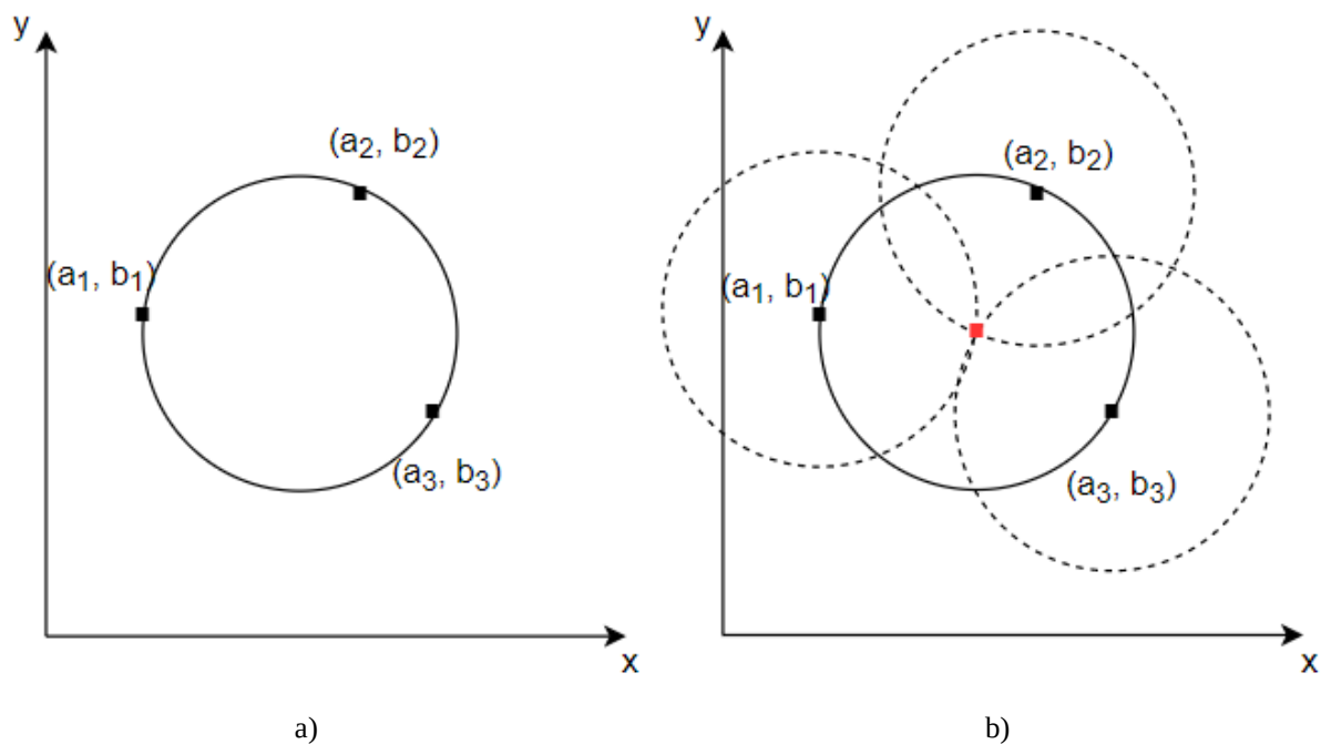
Slika 3.3. Proces upisivanja glasova u akumulacijsko polje a) izraženi rub u obliku kružnice, b) jedna dvodimenzionalna razina akumulacijskog polja za određeni radijus r
