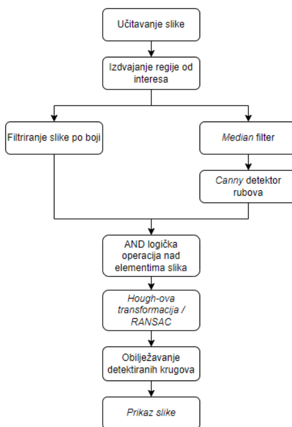
Slika 3.6. Blok dijagram algoritma za detekciju krugova pomoću Hough -ove transformacije ili RANSAC algoritma
