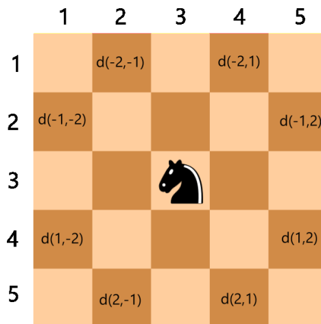
Sl. 5.8. Prikaz mogućeg kretanja skakača
