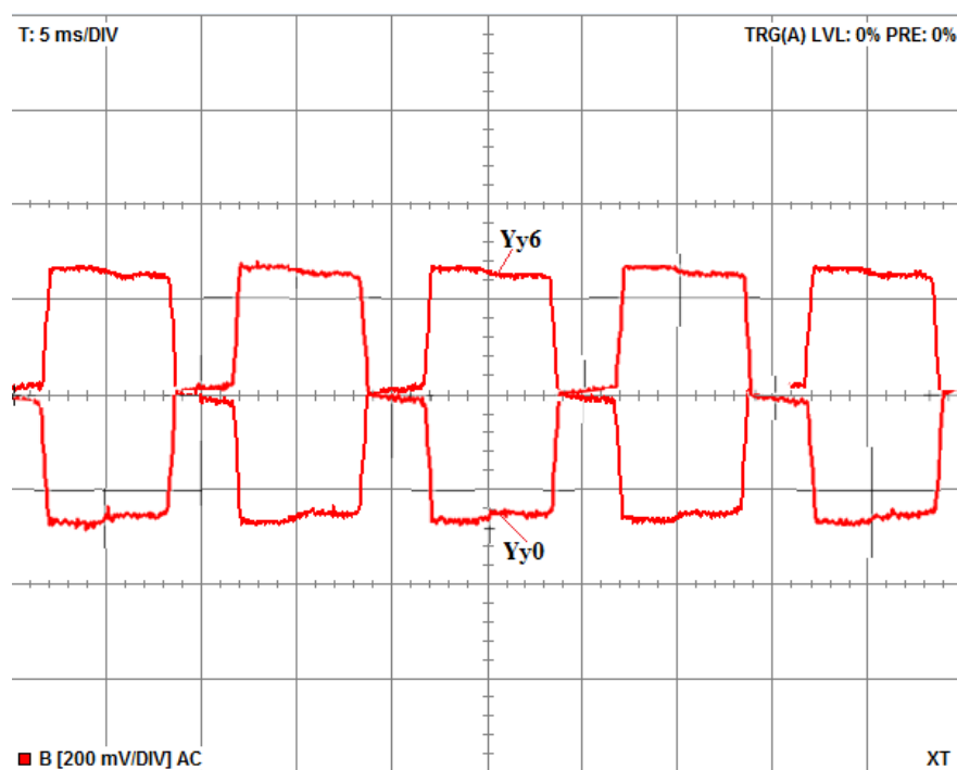
Slika 6.18. Usporedba linijske struje Yy0 i Yy6 grupe spoja
