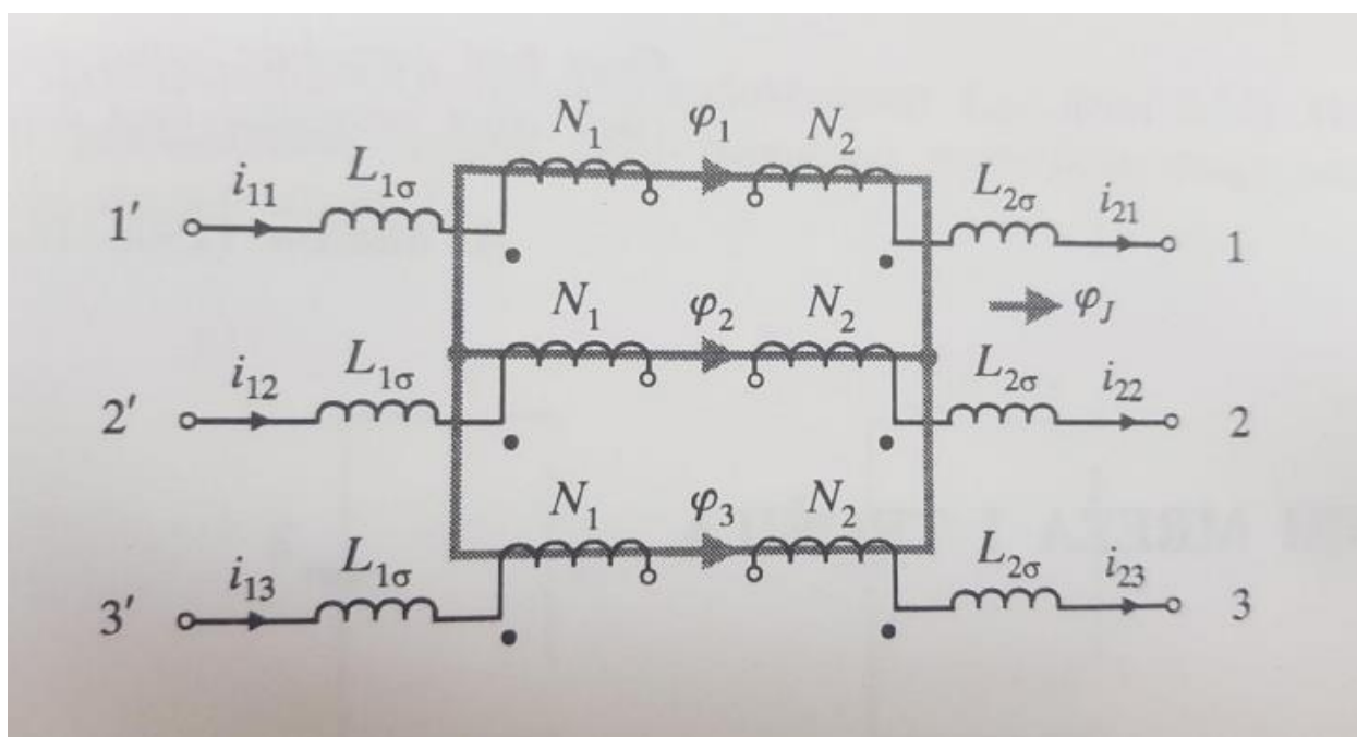
Slika 4.1. Model trofaznog transformatora[4]
