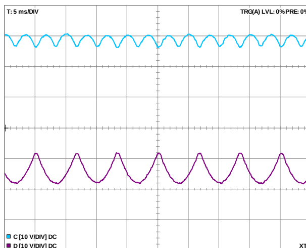
Izlazni napon ispravljača i napon na diodi
