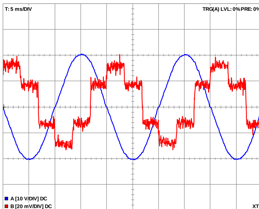
Slika 6.14. Valni oblici faznog napona (plavo) i fazne struje (crveno) (14V i 50Hz)
