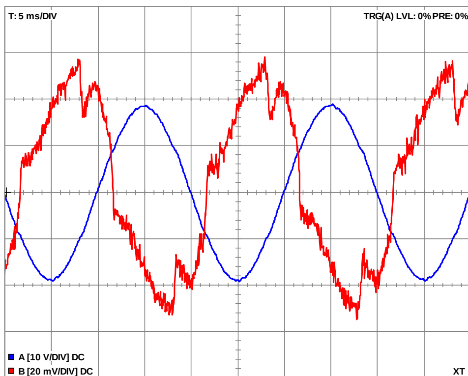
Slika 6.6. Valni oblik struje primara transformatora
