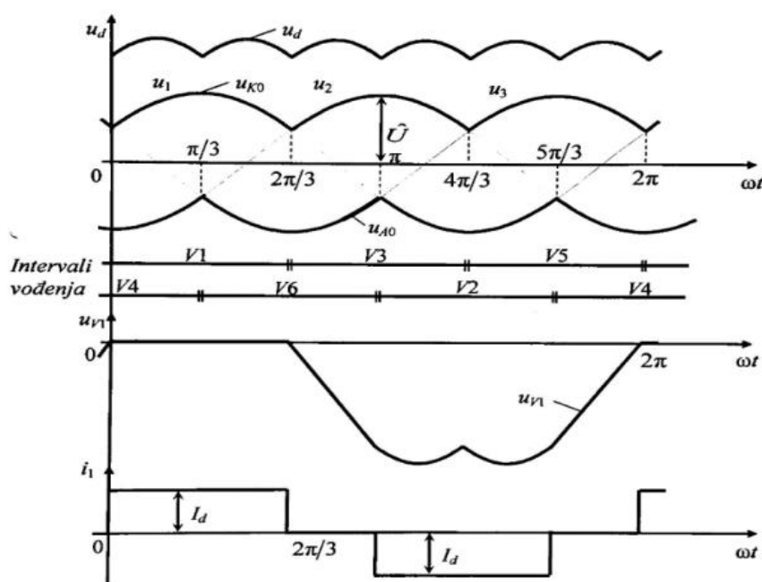
Slika 1.1. Karakteristični valni oblici induktivno opterećenog neupravljivog trofaznog mosnog spoja
