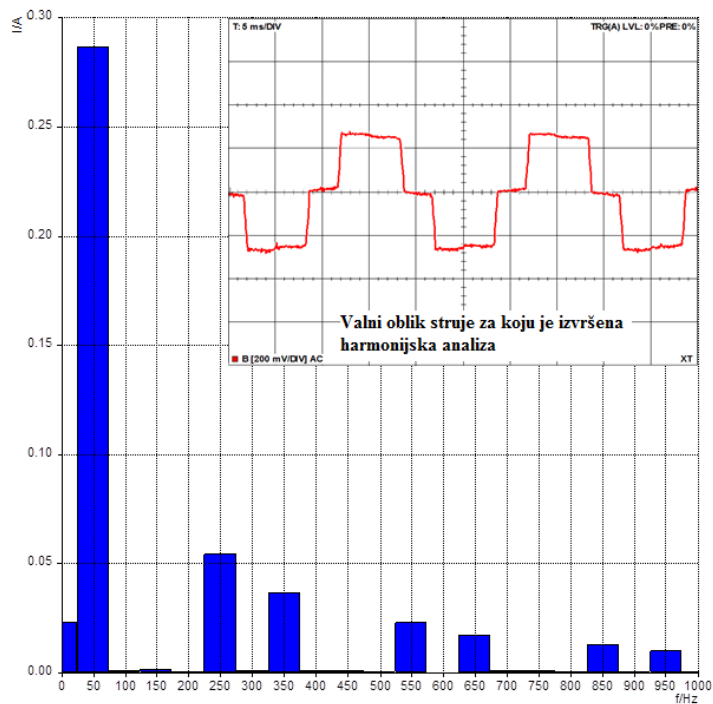
Slika 6.10. Harmonijska analiza faze struje i_1 sekundara transformatora u Yy0 spoju
