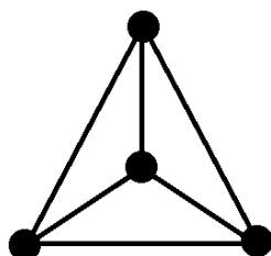
Slika 2.4 Potpuni graf K_4
