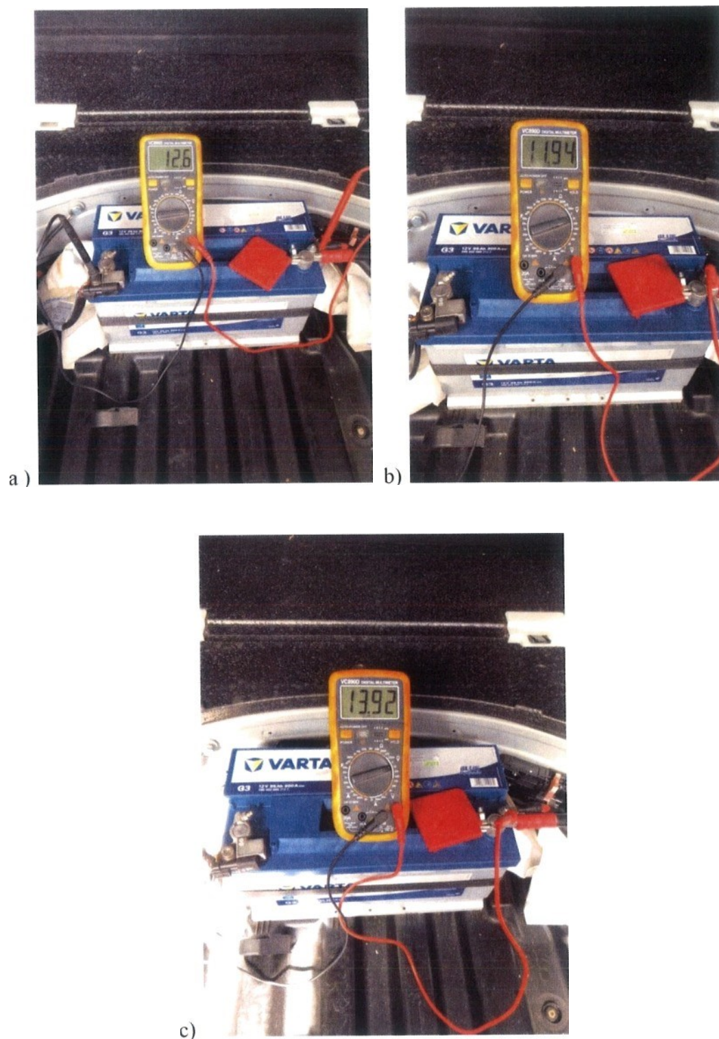
Slika 2.2.3 . Napon akumulatora u ,stanju mirovanja ( slika a),napon akumulatora firi pokretanju (slika b),napon akumulatora nakon u.staljenog stanja(slika c)
