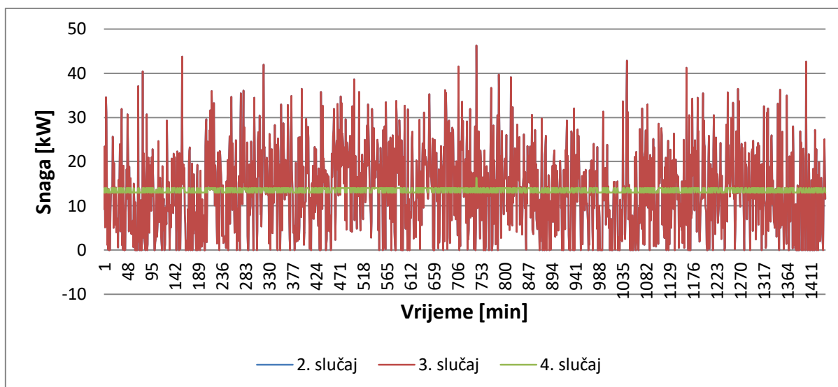
Slika 5.48. Tok ukupne radne snage na kraju izvoda za 3 slučaja.
