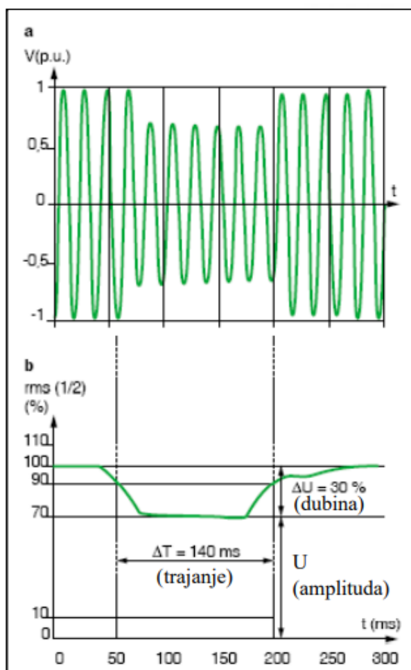
Slika 4.8. Naponski propad [8].
