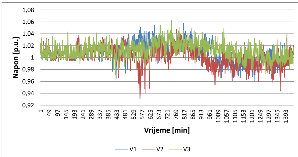
Slika 5.33. Napon na kraju izvoda.
