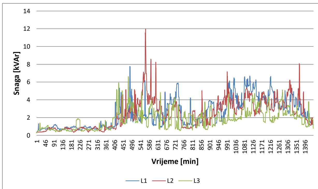
Slika 5.14. Tok jalove snage po fazama na početku izvoda.
