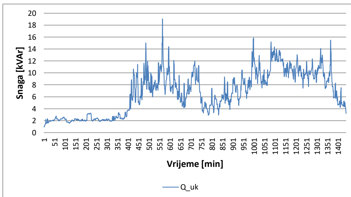
Slika 5.40. Tok ukupne jalove snage na početku izvoda.
