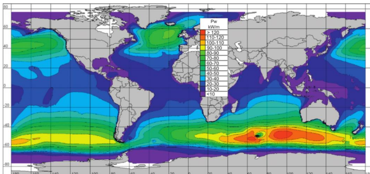
Slika 2.1. Globalna godišnja procjena srednje valne snage u \text{kW} / \text{m} u razdoblju od 10 godina. [1]
