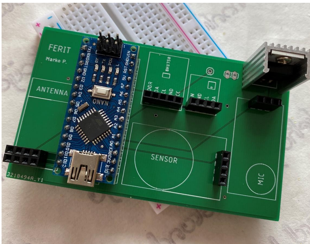
Slika 3.11. Izradeni PCB
