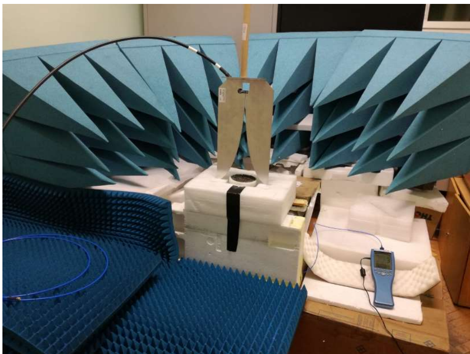
Slika 2.2. Tretiranje sjemeni električnim poljem u rasponu od 0,8 do 8 GHz u Laboratoriju za VF mjerenja Fakulteta elektrotehnike, računarstva i informacijskih tehnologija u Osijeku
