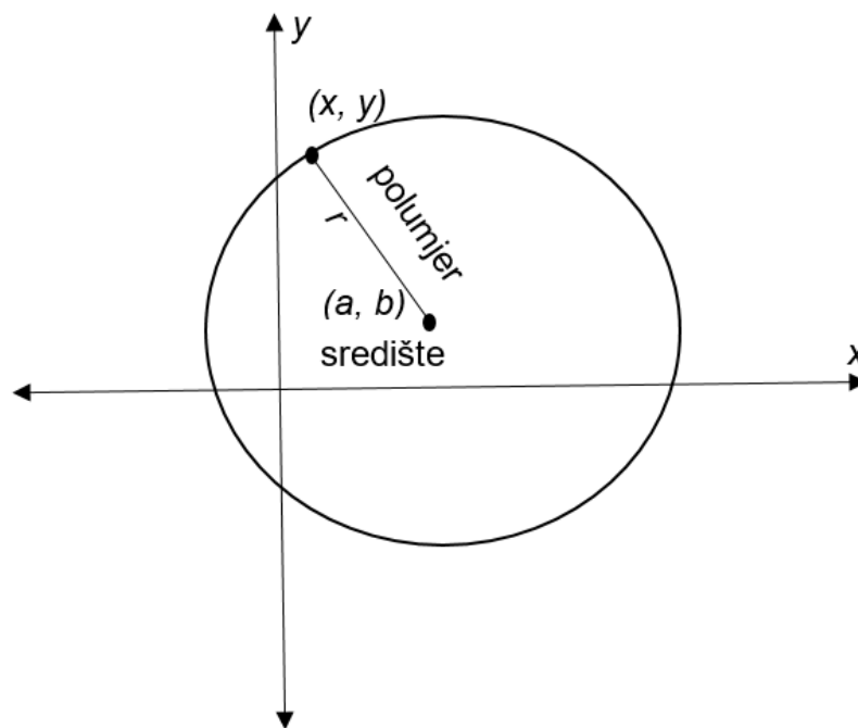
Slika 3.3. Houghova transformacija
