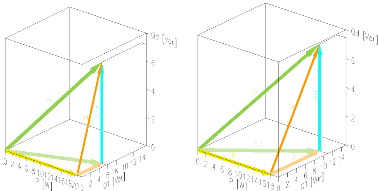
Slika 4.7. Trodimenzionalni prikaz komponenata snage za \alpha=15^\circ (lijeva slika) i 25^\circ (desna slika).
