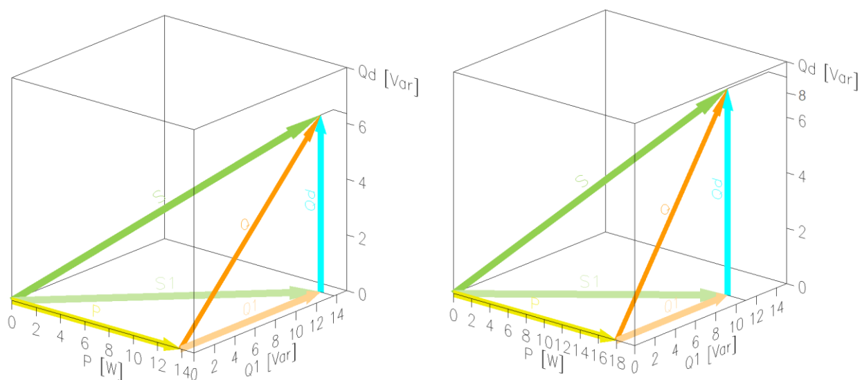
Slika 5.2. Trodimenzionalni prikaz komponenata snaga za \alpha=45^\circ , punoupravljivi (lijeva slika) i poluupravljivi (desna slika).
