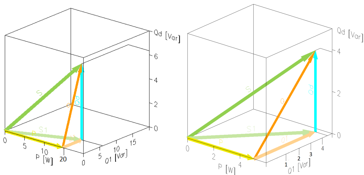
Slika 4.13. Trodimenzionalni prikaz komponenata snage za \alpha=15^\circ (lijeva slika) i \alpha=75^\circ (desna slika).
