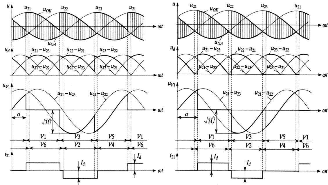
Slika 3.5. Karakteristični valni oblici poluupravljivog ispravljača za \alpha < 60^\circ (lijeva slika) i 60^\circ < \alpha < 90^\circ (desna slika), [6].
