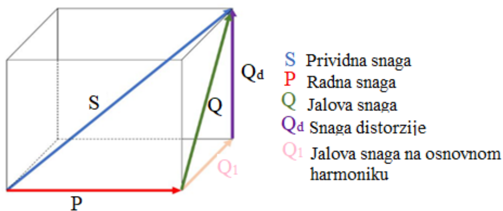
Slika 4.6. Trodimenzionalni prikaz komponenata snage, [6].
