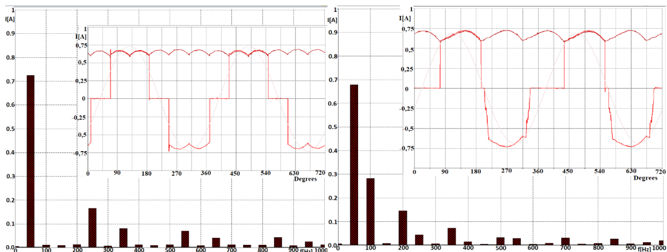
Slika 5.1. Prikaz harmonika za \alpha=45^\circ , punoupravljivi (lijeva slika) i poluupravljivi (desna slika).
