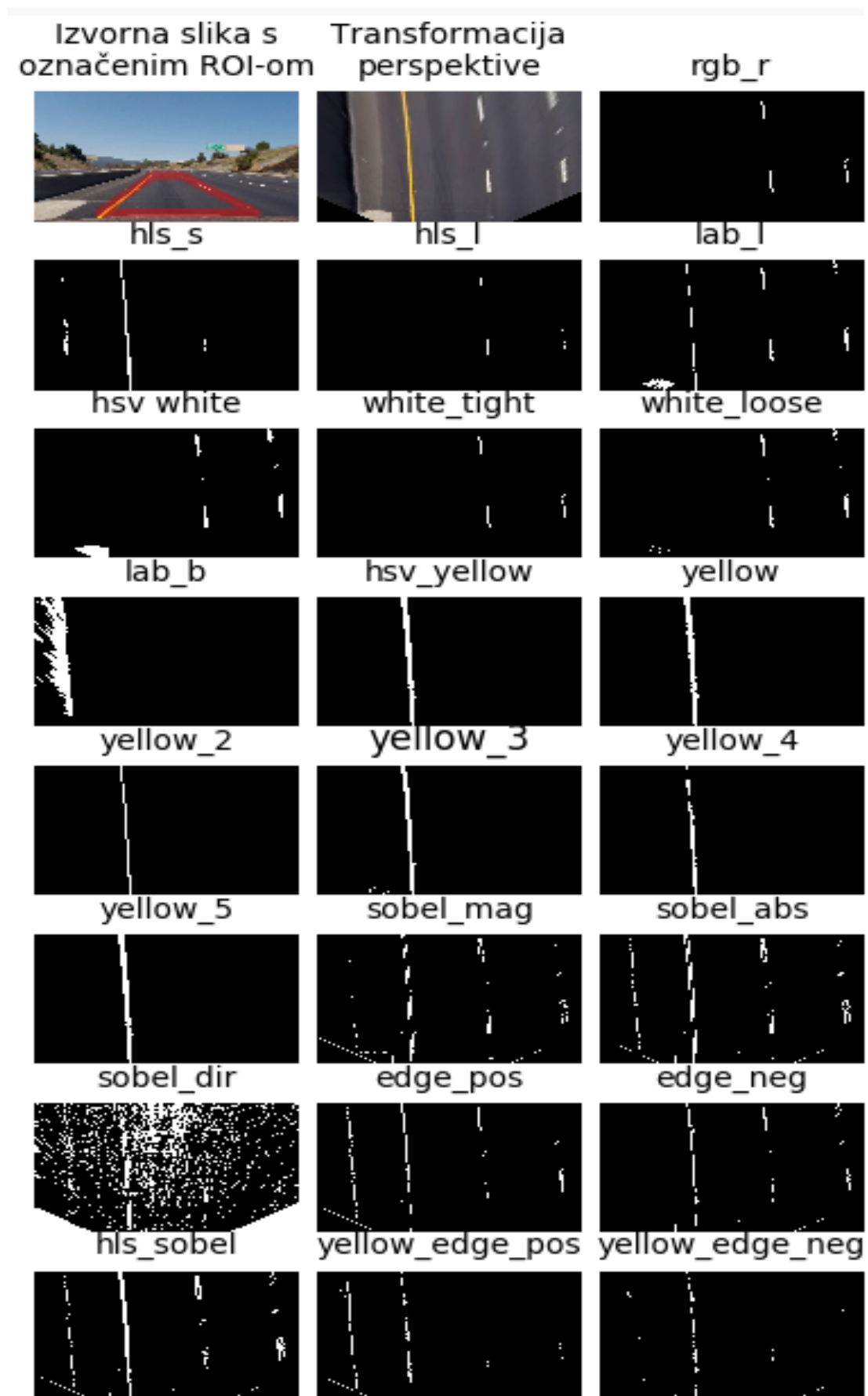
Slika. 3.7. Prikaz svih kreiranih binarnih slika s njihovim nazivima nakon primjene odgovarajućih filtara.
