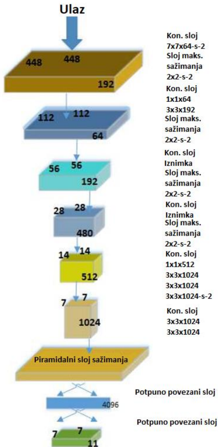
Slika 2.3. Arhitektura mreže [12]
