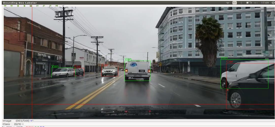
Slika 3.5. OpenLabeling alat
