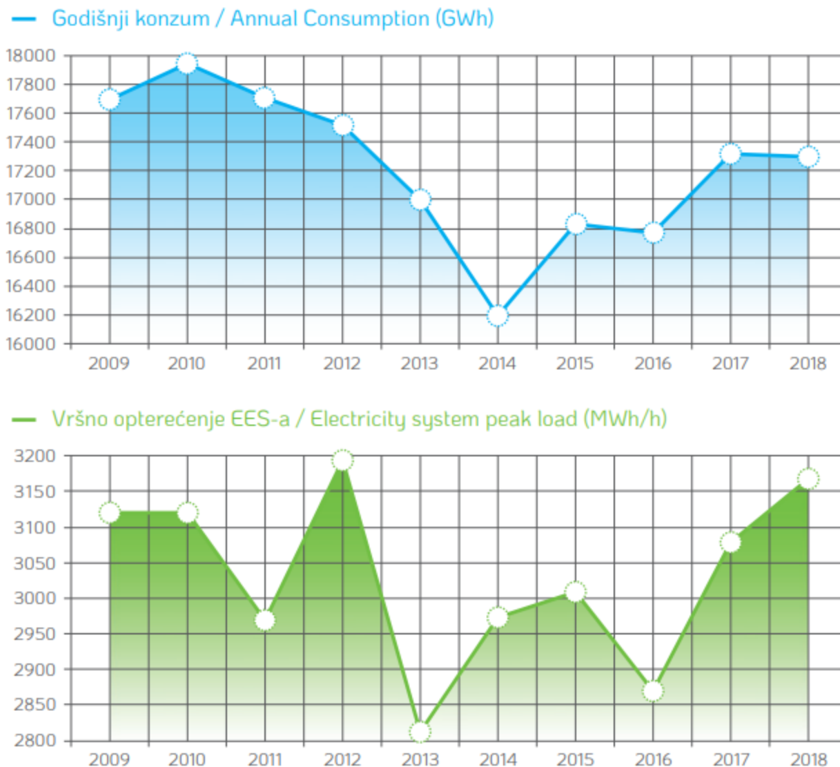
Sl. 3.2. Godišnja potrošnja na prijenosnoj mreži i vršno opterećenje u posljednjih 10 godina [9]
