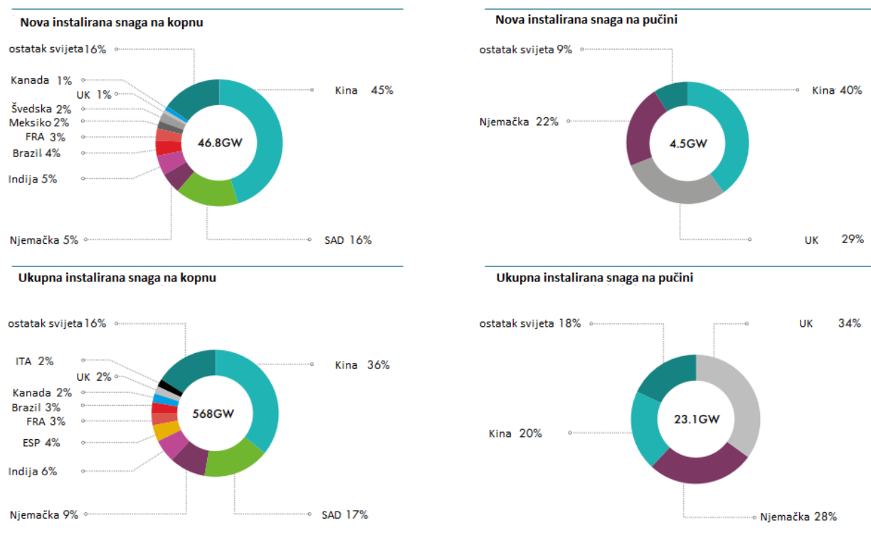
Sl. 2.7. Instalirane snage na kopnu i pučini za 2018. godinu [3]
