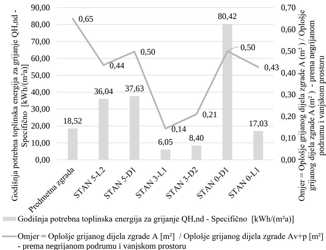
Graf 4.22. Usporedba geometrijskih podataka i podataka o energetskeim svojstvima – novo stanje.
