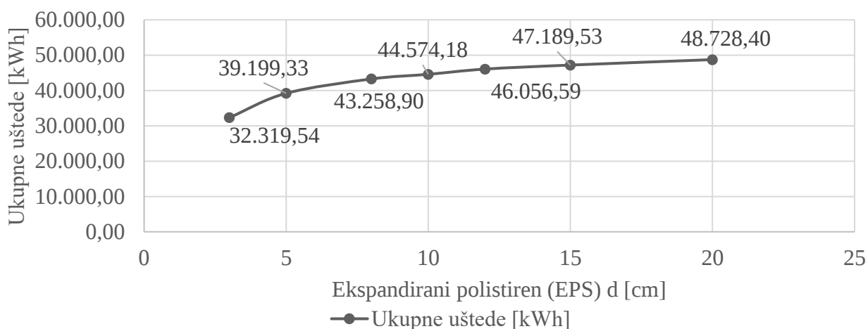
Graf 4.9. Prikaz veze između uštede u energiji za grijanje u kWh i debljine toplinske izolacije u cm.
