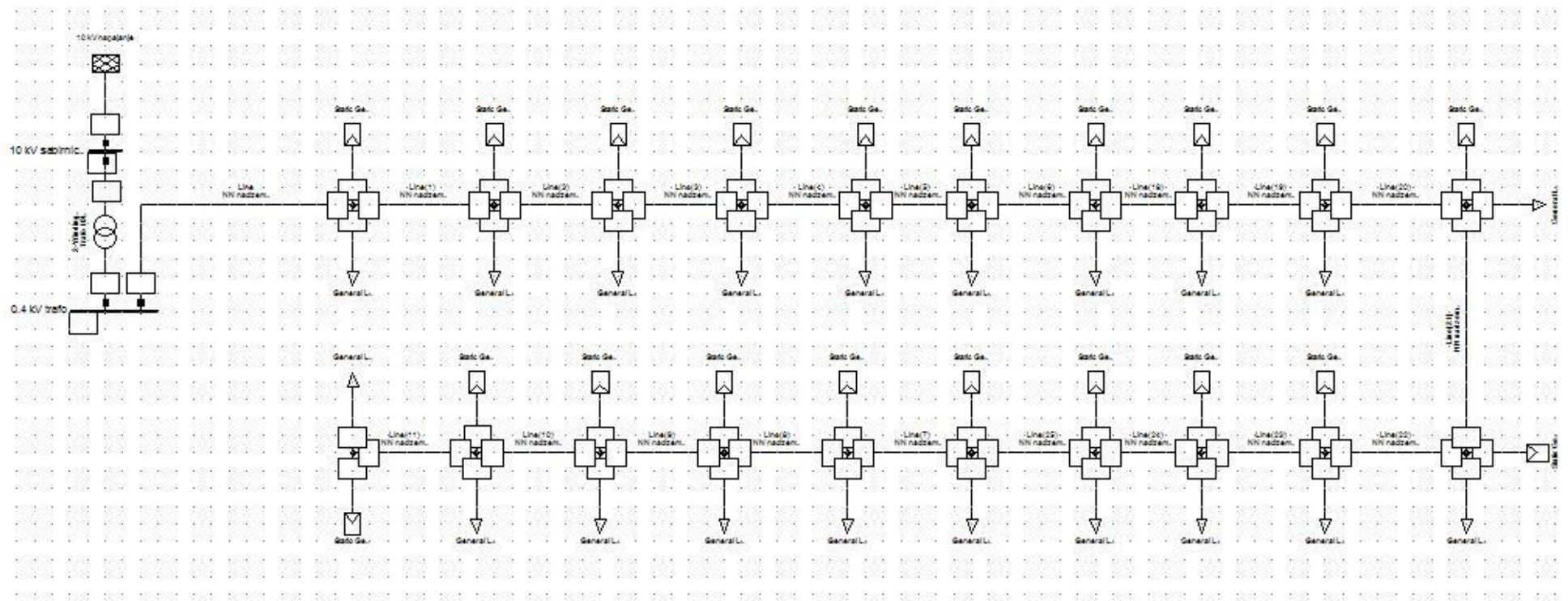
Sl.4.1 Računalni model koji predstavlja tipičan dio rezidencijalne distribucijske mreže, a pretpostavka je da svaka kuća ima instaliranu FN elektranu.
