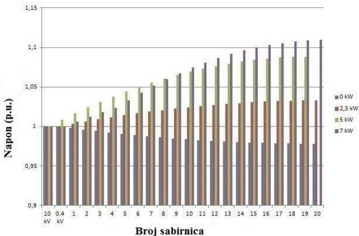
Sl.4.4. Profili napona za različite razine proizvodnje fotonaponskih sustava, dok je potrošnja u stambenim jedinicama jednaka 1 kW
