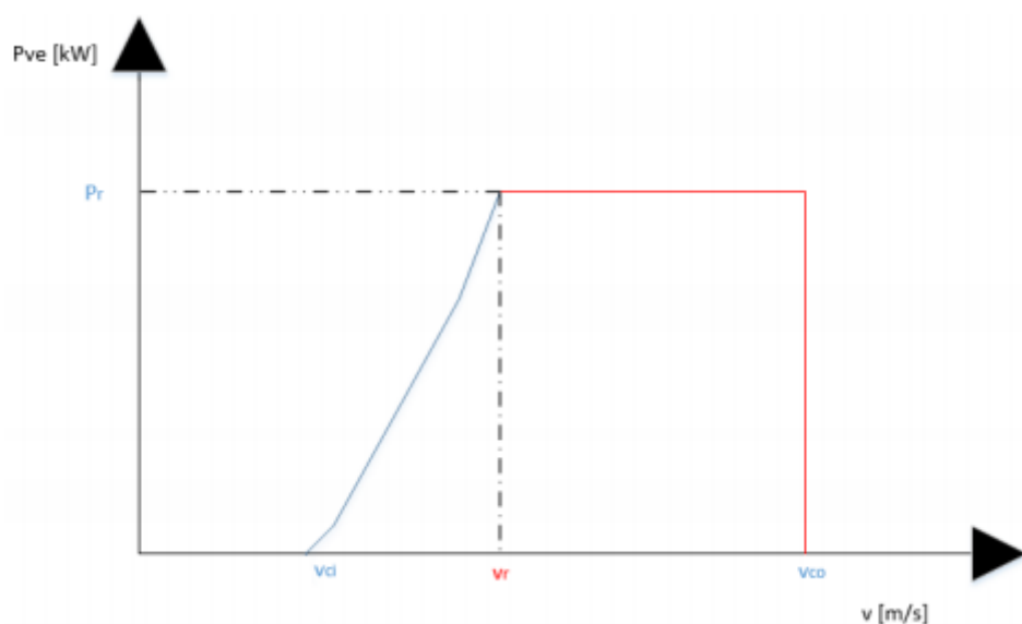
Sl. 2.11. Krivulja snage i tri ključne brzine [3]
