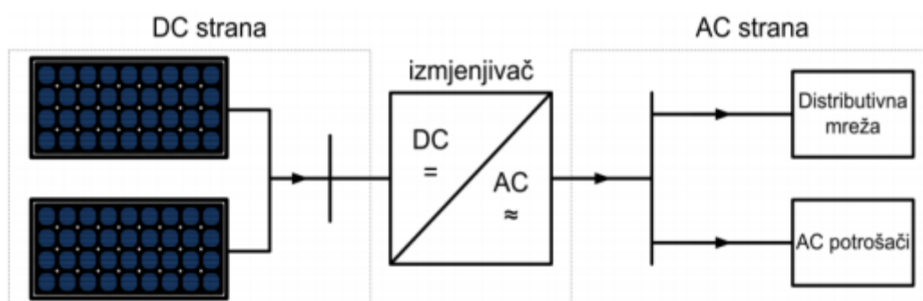
Sl.2.18. Potpuno neizravni priključak FNE putem istosmjernog pretvarača napona (MPPT, Chopper) i izmjenjivača [9]
