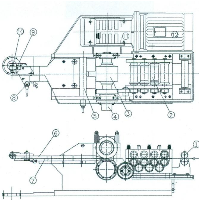
Slika 3.4 – Dijelovi stroja
