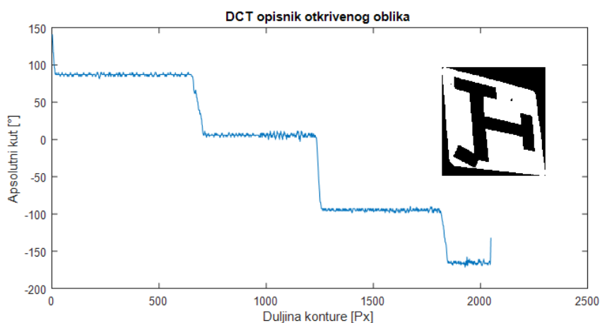
Slika 3.28. DCT opisnik distorziranog znaka slijepe ulice
