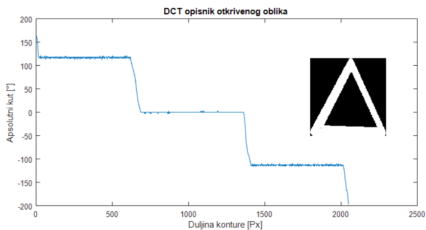
Slika 3.40. DCT opisnik distorziranog znaka „zavoj ulijevo“
