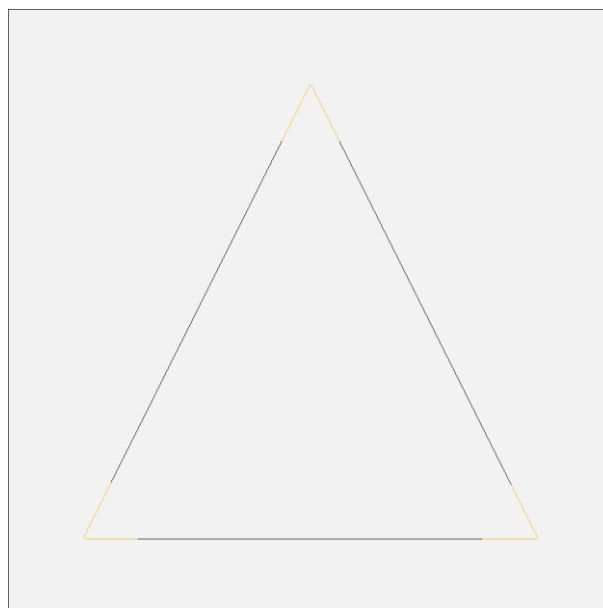
Slika 3.4. Jednakokračan trokut s označenim kutovima i stranicama
