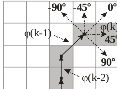
b) Traženje piksela u (k+1)-om koraku.
