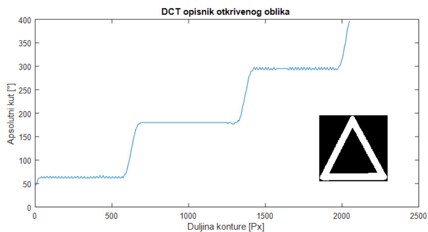
Slika 3.39. DCT opisnik za znak „zavoj ulijevo“ fotografiranog iz daljine
