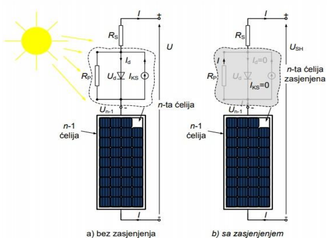
Slika 3.34. FN moduli sa i bez zasjenjenja [10]
