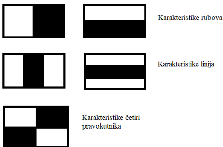
Sl. 2.2. Izgled Haarovih karakteristika [1]
