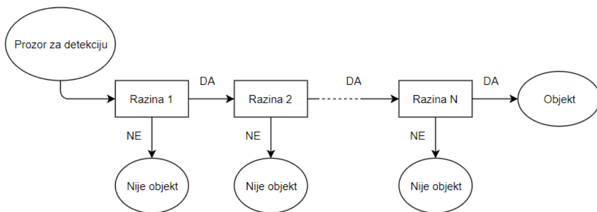
Sl. 2.3. Način rada kaskade klasifikatora [1]
