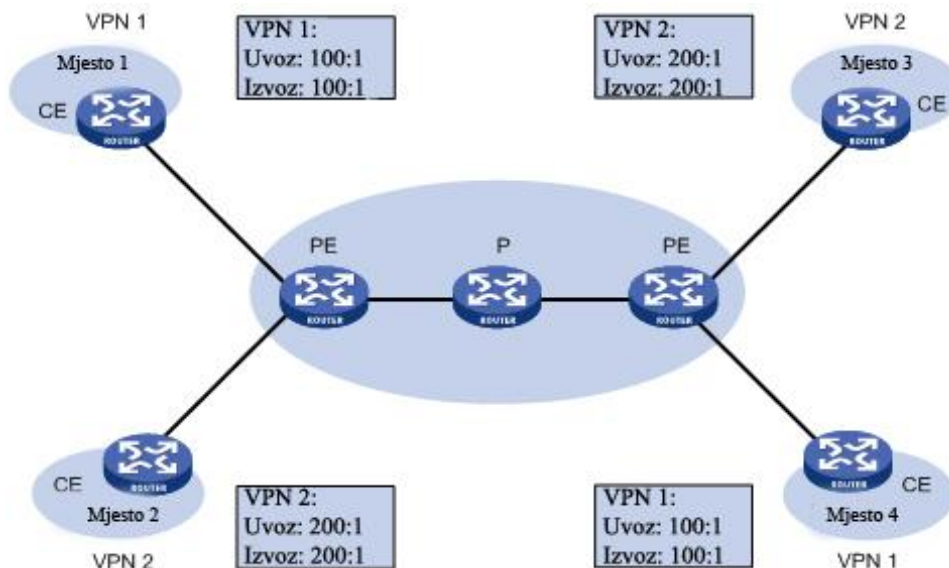
Slika 5.4. Route target [46]
