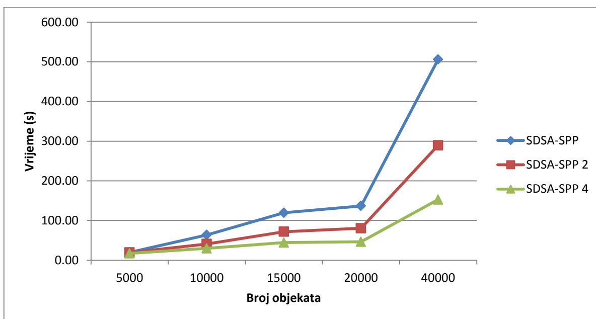
Slika 5.31 Vremena izvođenja serijskih i paralelnih algoritama korištenjem osnovnih parametara prikazanih u tablici 5.1
