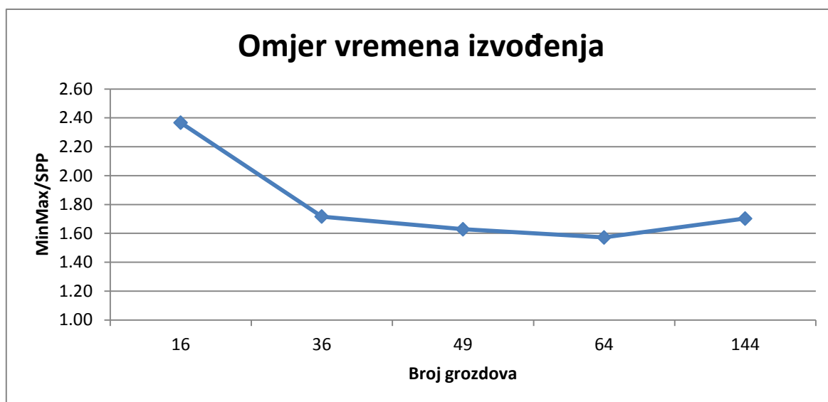
Slika 5.7 Omjer vremena izvođenja algoritama MinMax i SPP za različit broj grozdova
