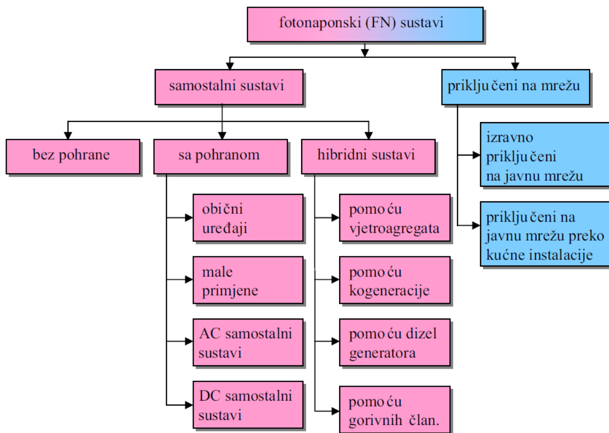
Sl 2.1. Osnovna podjela fotonaponskih sustava [1, str. 369].
