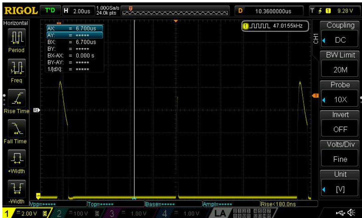
Slika 3.2.8-Signal poslije komparatora usljed djelovanja induktiviteta za kondenzator kapaciteta 56pF
