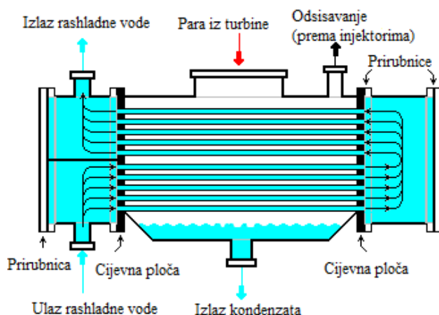
Sl.2.10. Shematski prikaz vodom hlađenog kondenzatora [10].
