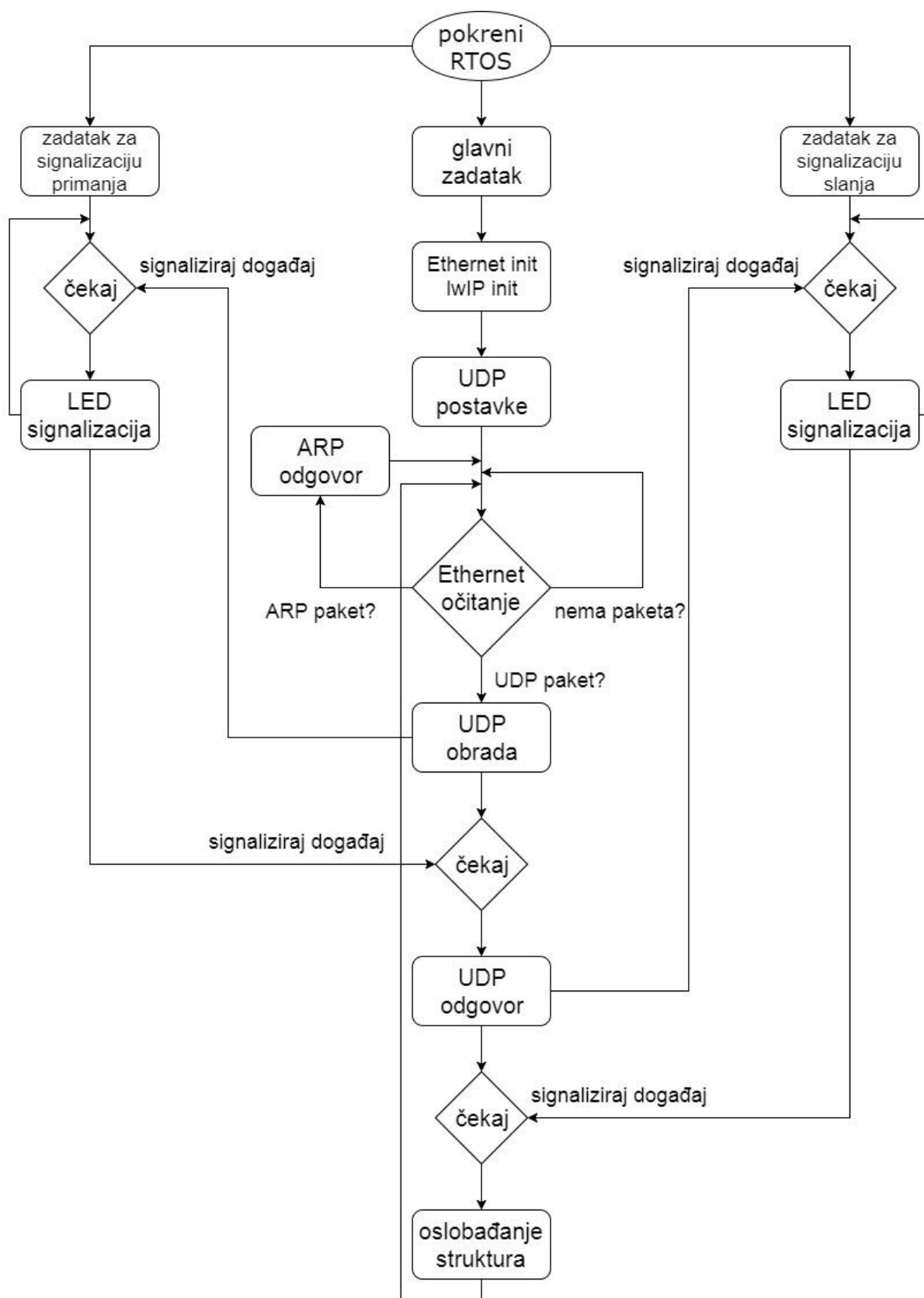
Slika 3.12. Blokovski dijagram algoritma UDP poslužitelja
