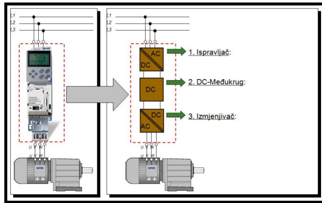
Slika 3.3. Shema frekvencijskog pretvarača [10]
