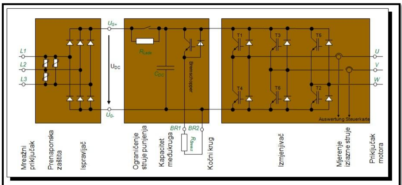
Slika 3.4. Konfiguracija energetskog pretvarača [10]
