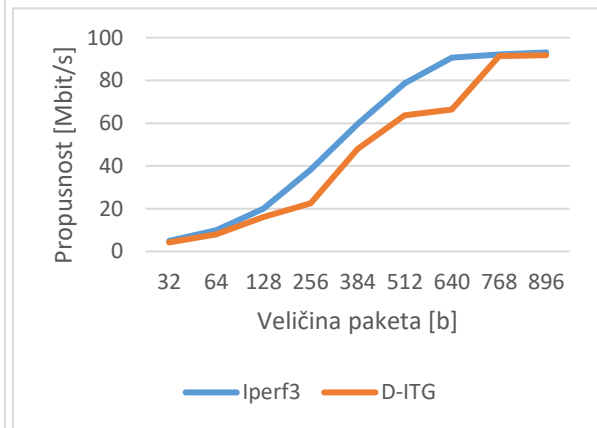
Slika 5.8. UDP propusnost
