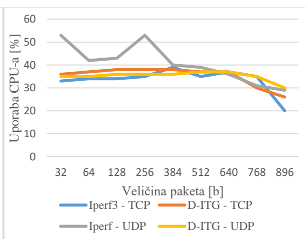
Slika 5.10. Uporaba CPU-a
