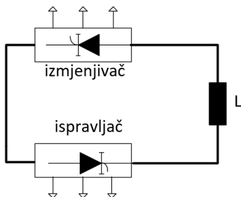
Slika 4.10. Pretvarač sa strujnim izvorom[1]
