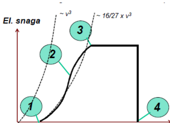
Slika 2.4. Krivulja snage vjetroatregata [1]
