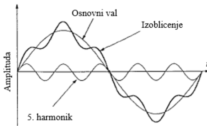
Slika 3.6. Izoblićeni sinusni val [10]
