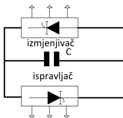
Slika 4.11. Pretvarač s naponskim izvorom [1]
