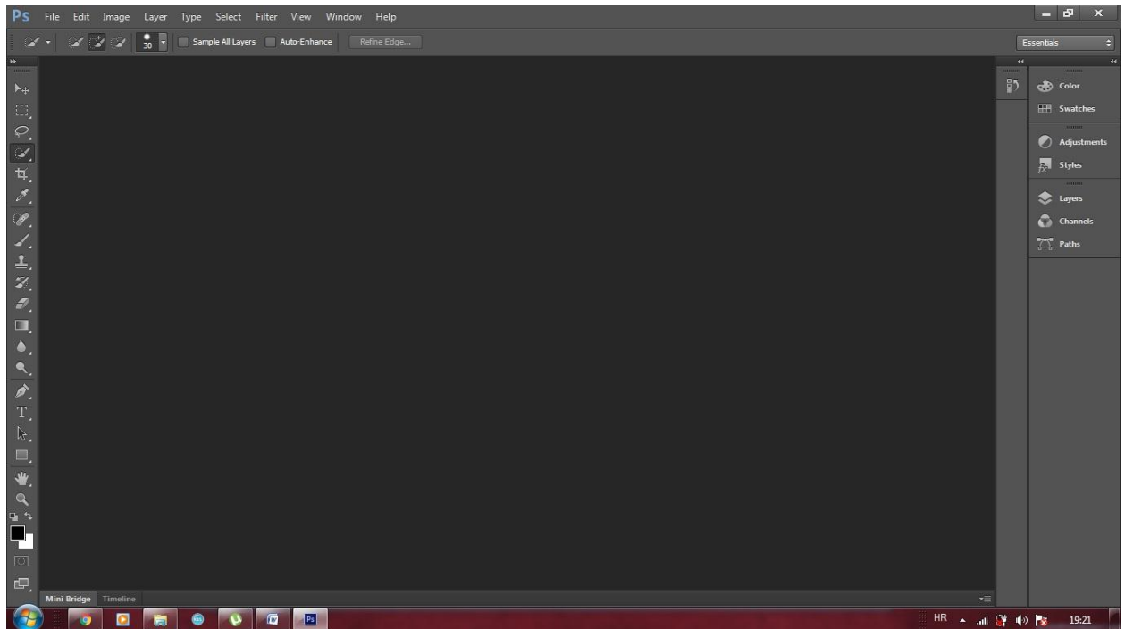
Slika 3.2 Sučelje Photoshopa
