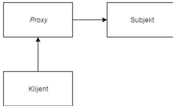
Slika 2.11. Struktura Proxya
