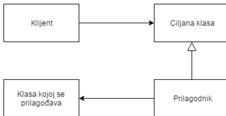
Slika 2.5. Struktura Prilagodnika
