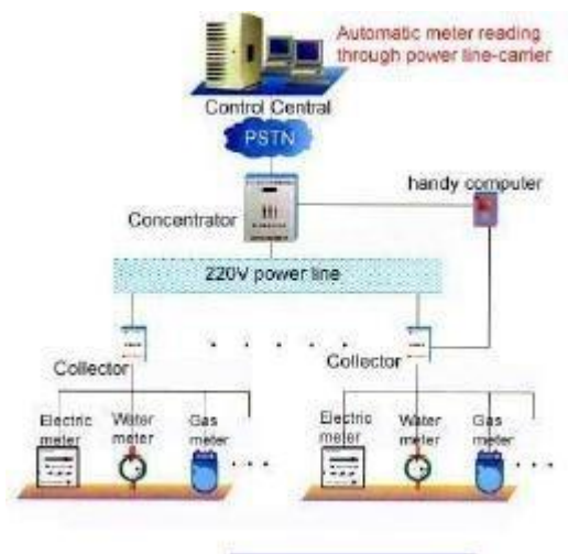
Slika 3.1. Koncept daljinskog očitavanja korištenjem PLC tehnologije
