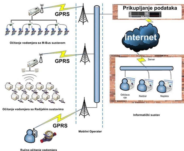
Slika 3.6. Daljinsko očitavanje potrošnje vode preko GPRS komunikacije
