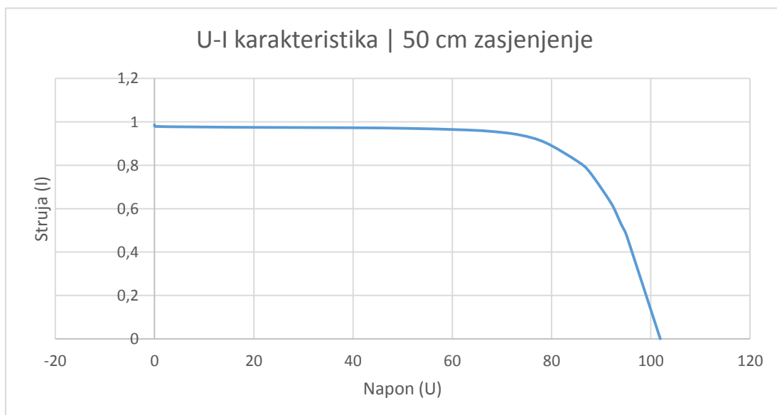
Slika 5.19. U-I karakteristika pri zasjenjenju fotonaponskog modula SOLAR FRONTIER SF-150 od 50 cm.
