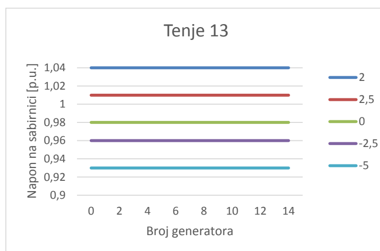
Slika 3.3. Utjecaj broja generatora na napon u niskonaponskom izvodu Tenja 13
