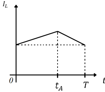
Sl. 3.4. Valni oblik struje induktiviteta
