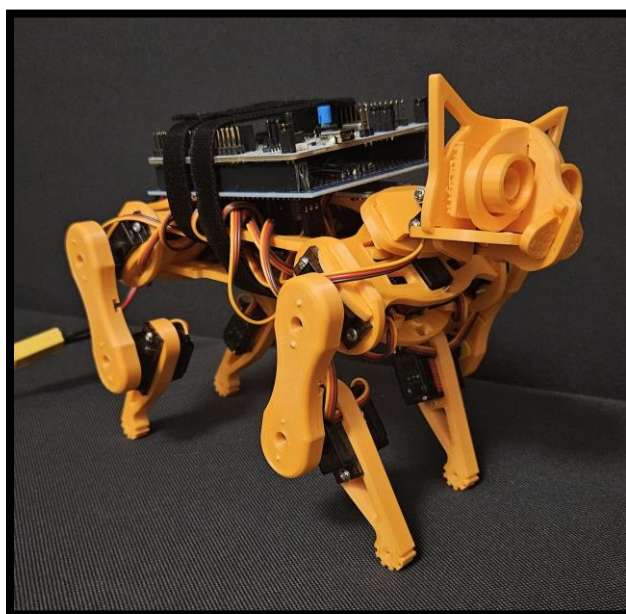
Slika 5.8. Sastavljeni model robota Nybble
