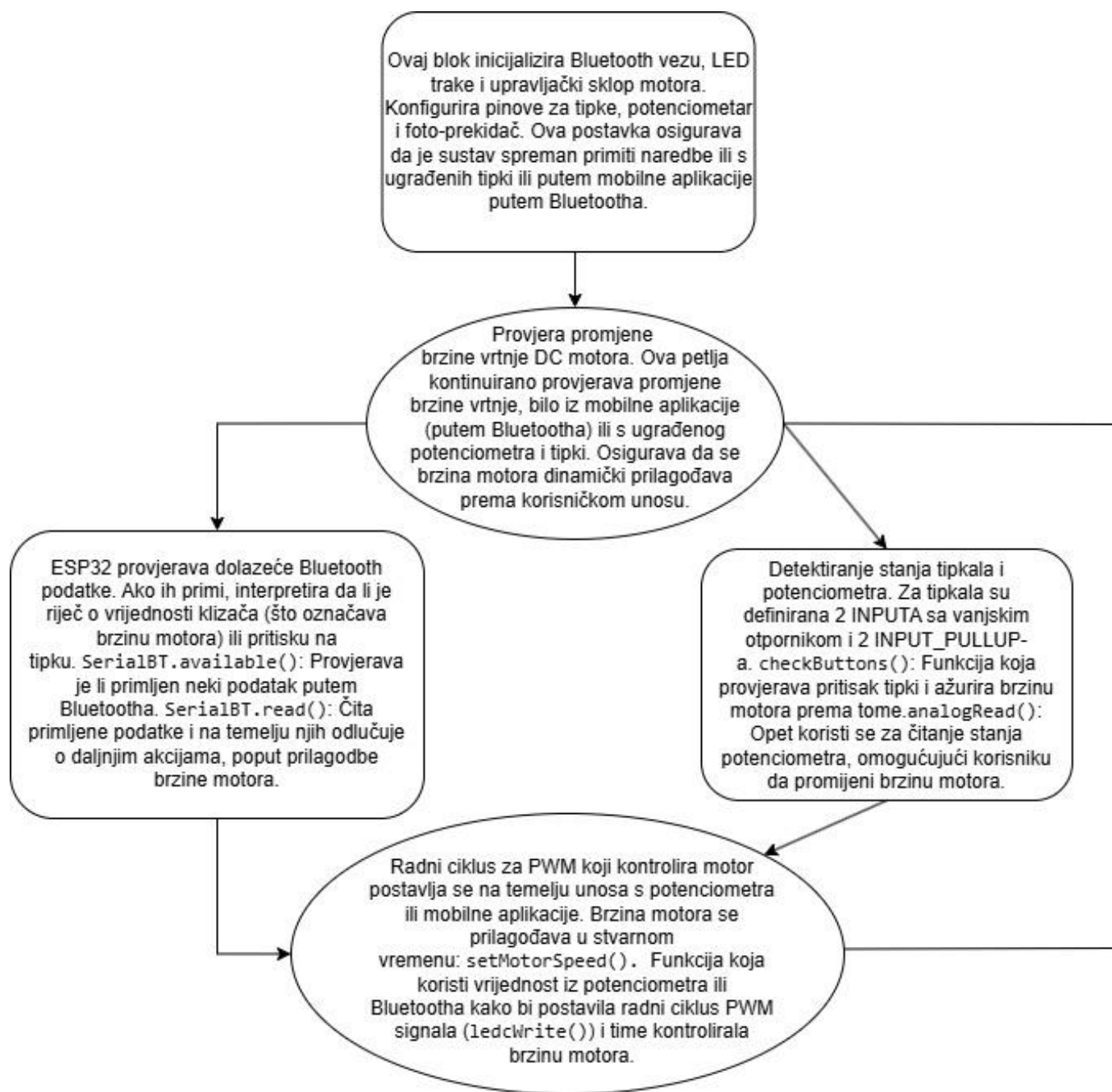
Slika 3.7. Prikaz blok dijagram toka realiziranog programskog koda
