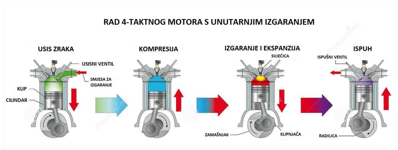
Slika 2.2. Prikaz 4-taktnog ciklusa u cilindru [6]
