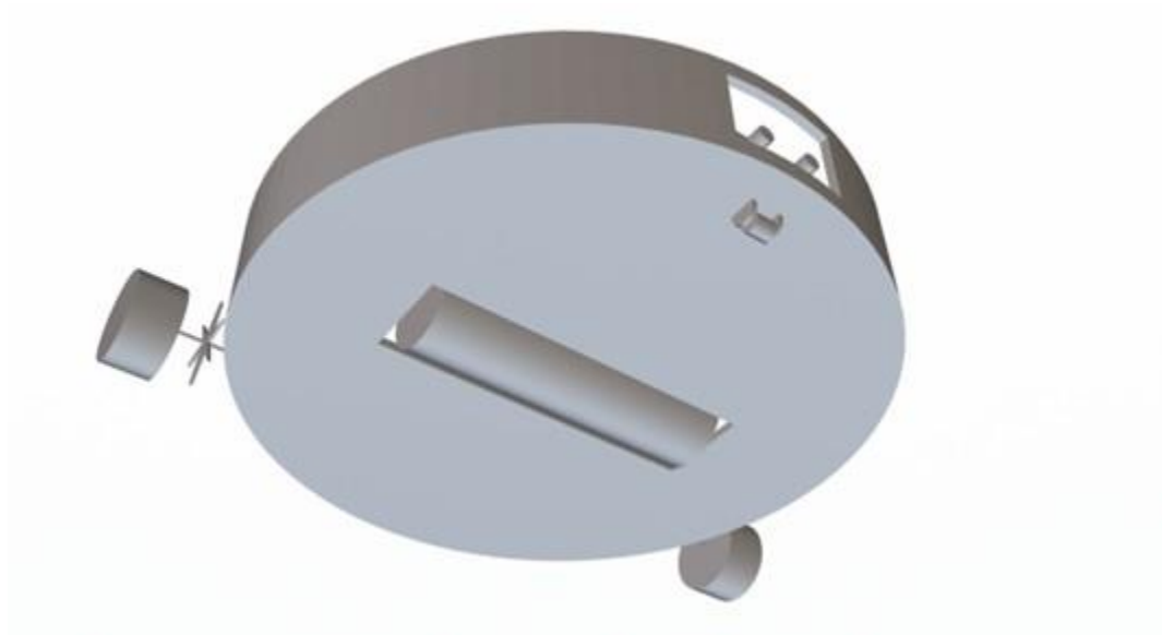
Slika 2.6. Prikaz 3D modela kojim je predstavljeno rješenje problema pozicioniranja četke kako bi ista dopirala do podne podloge.
