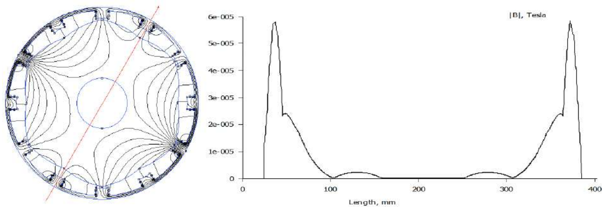
Slika 4.10. Prikaz raspodjele magnetske indukcije duž promjera senzora (pri struji uzbudnog namota od 0.0083 mA)
