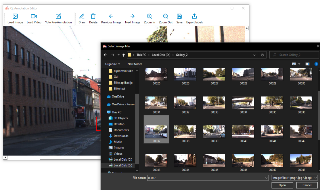
Slika 4.8. Verifikacija prikaza dijaloškog okvira s navigacijom i filtrom formata za dodavanje slike u postojeću projektnu galeriju
