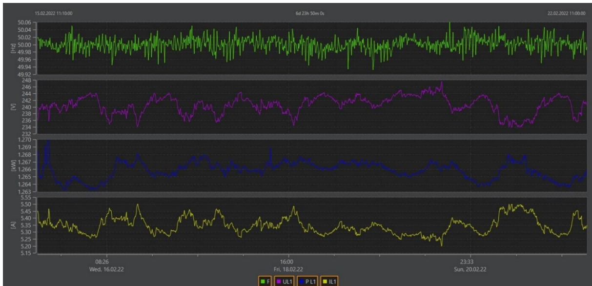
Slika 6.19. Promjena frekvencije, napona, snage i struje u mjerenom periodu u drugom tjednu mjerenja
