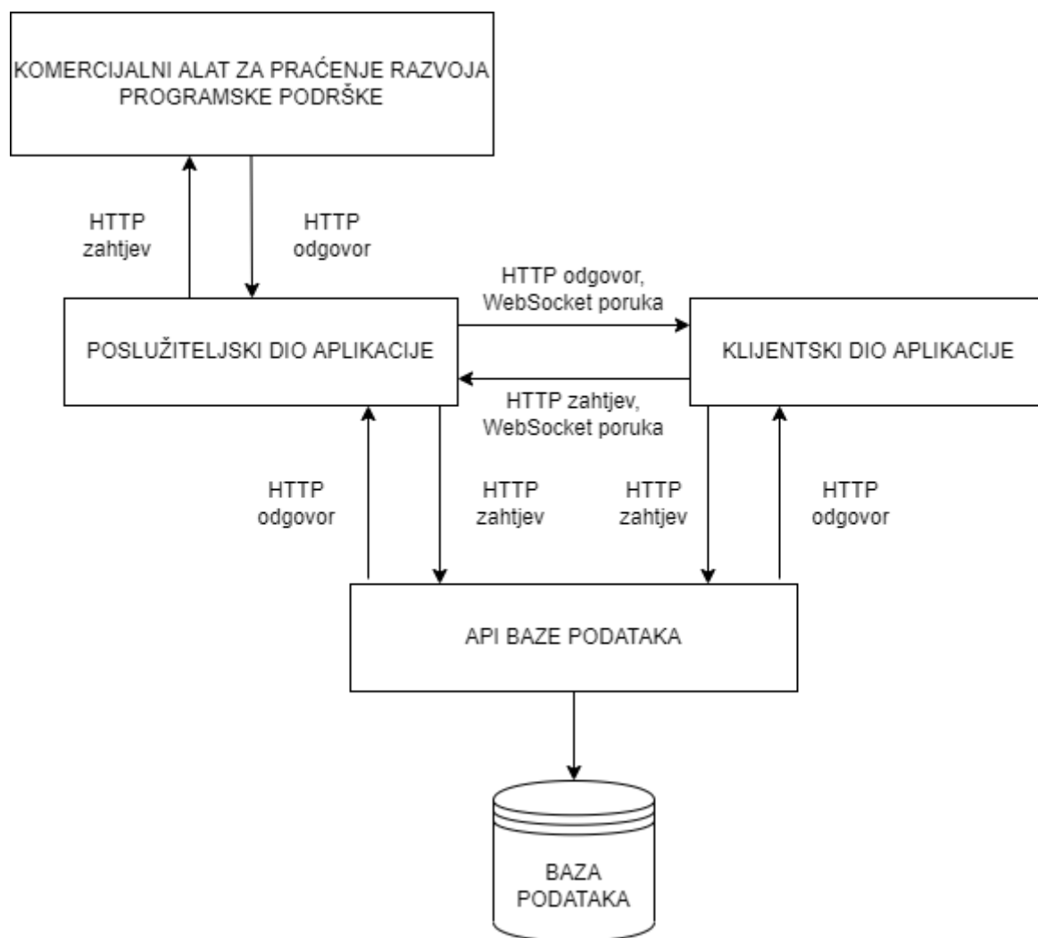
Slika 3.1. Arhitektura aplikacije.
