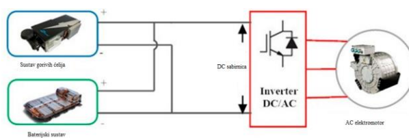
Slika 3. 12. Topologija 1
