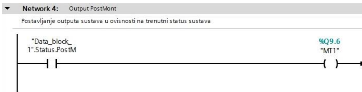
Slika 3.23 Postavljanje izlaza sustava MT1 u ovisnosti na trenutni status sustava
