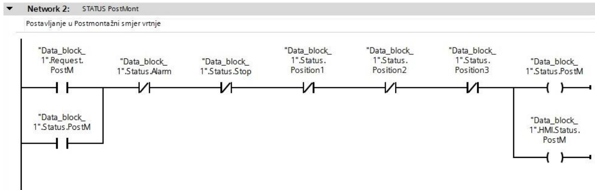
Slika 3.21 Postavljanje statusa u postmontažni smjer vrtnje
