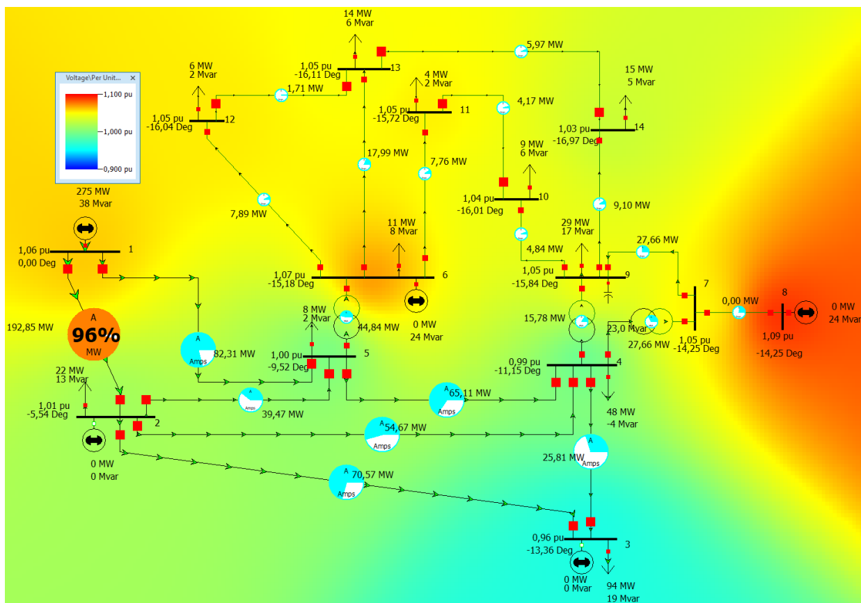
Sl.5.12. Naponske prilike u sustavu
