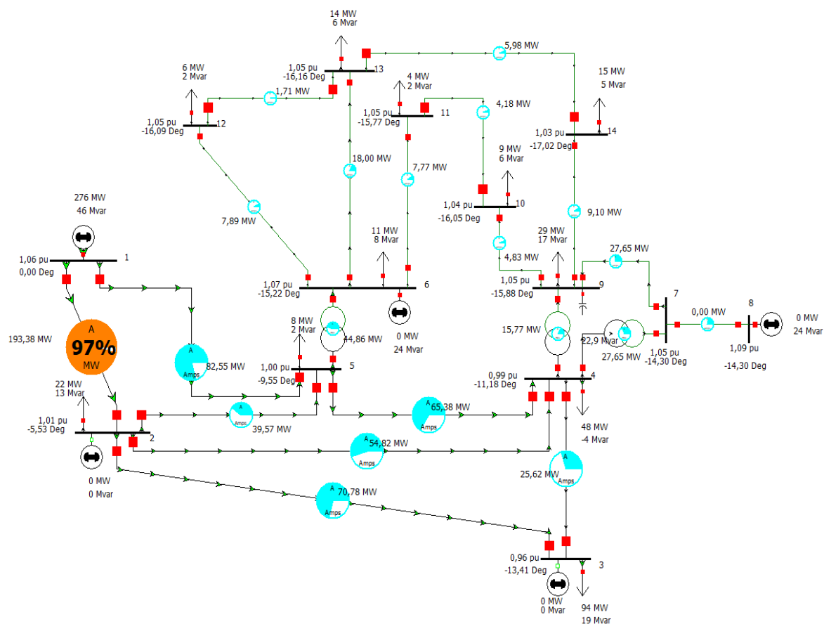
Sl.5.1. IEEE testna mreža sa 14 sabirnica na kojoj je rađena simulacija
