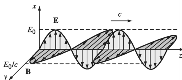
Slika 5.1: Elektromagnetski val u vakuumu [3]
