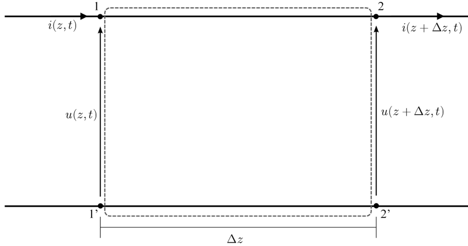
Slika 5.5: Objašnjenje primjene jednadžbe (5-8) — prikazana je petlja na koju se primjenjuje Faradayev zakon
