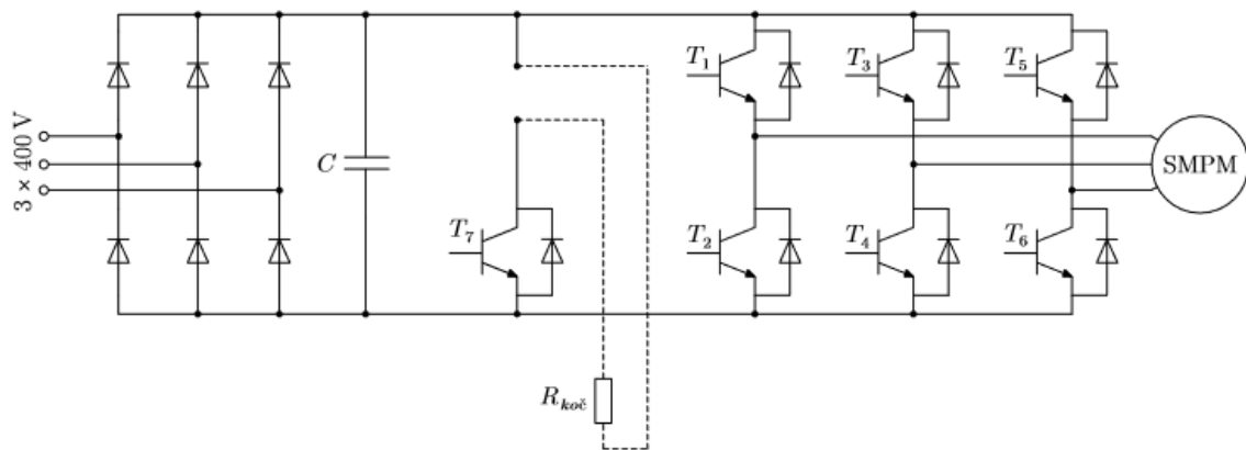
Sl. 4. 3. Shema pretvarača napona i frekvencije
