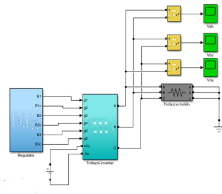
Sl. 5. 1. Vektorsko upravljanje pomoću PWM-a
