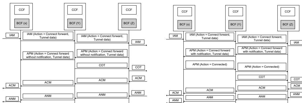
Slika 14. Ubrzano prospajanje unaprijed bez i s potvrdom o konekciji [10]
