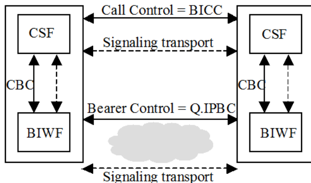
Slika 11. Mehanizam tuneliranja [10]
