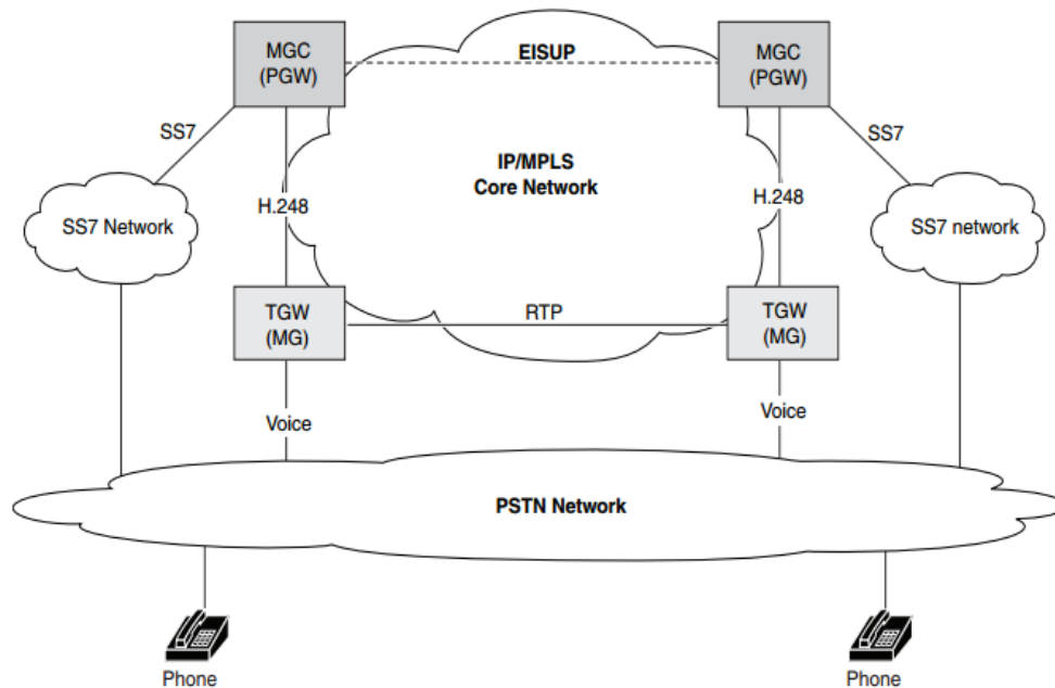
Slika 20. H.248 protokol u SS7 mreži [12]
