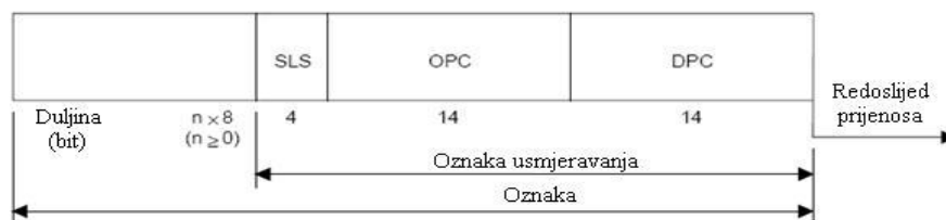
Slika 8. Struktura oznake usmjeravanja
