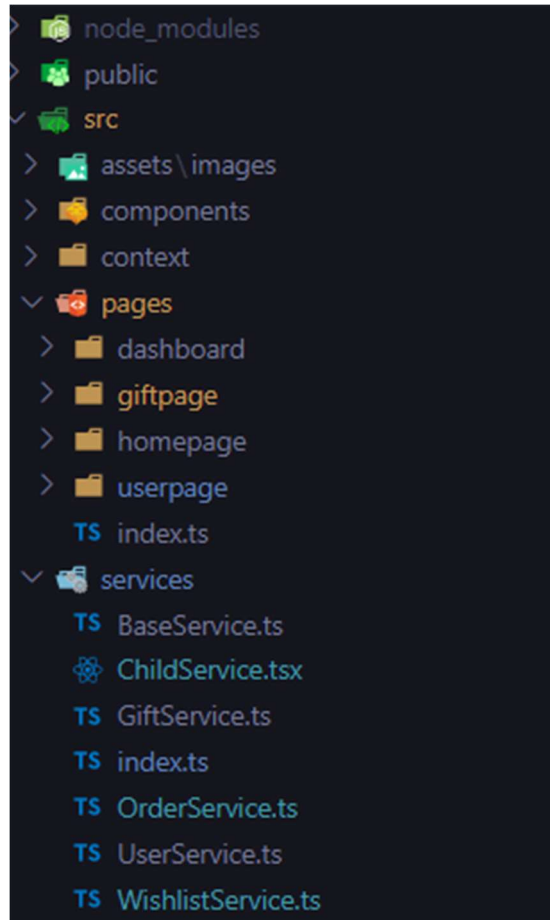
Slika 5.3. Struktura direktorija.
