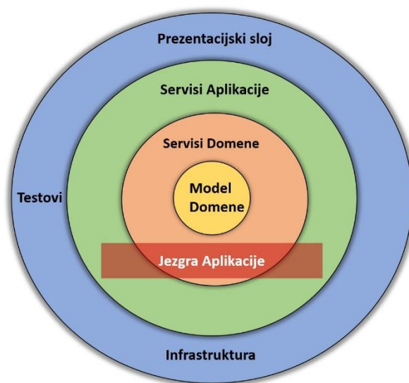
Slika 4.6. Onion arhitektura
