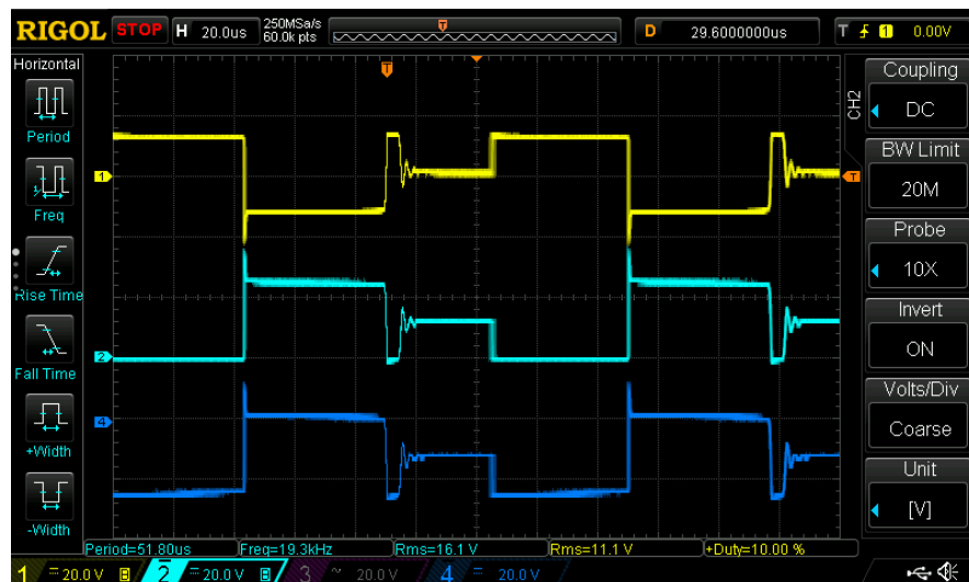
Slika 5.4. Valni oblici napona u_L , u_{T1} i u_{D1} u diskontinuiranom režimu rada
