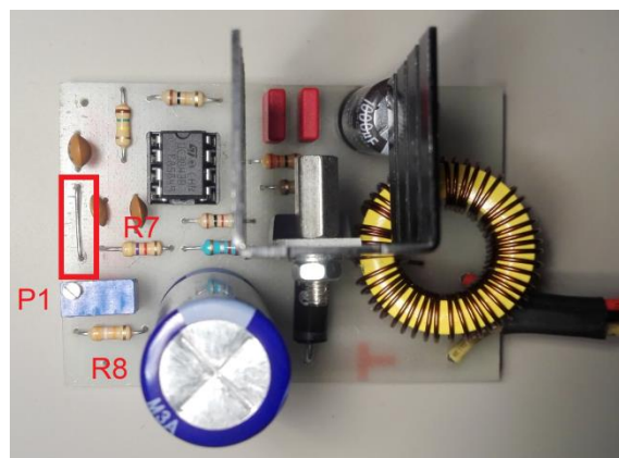
Slika 4.7. Izgled završenog sklopa
