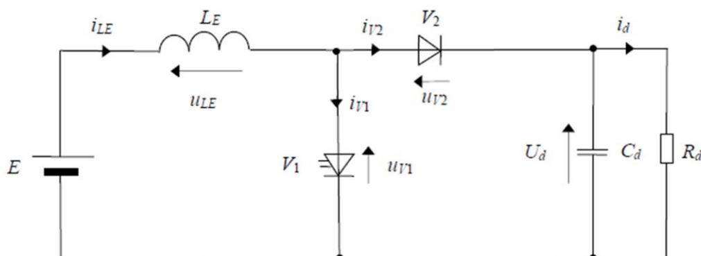
Slika 3.1. Nadomjesna shema uzlaznog pretvarača napona
