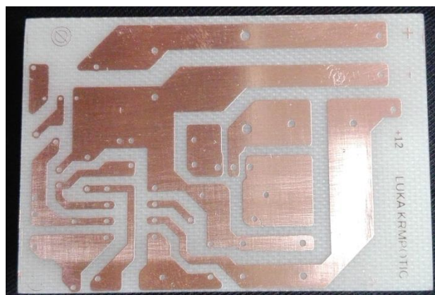
Slika 4.5. Tiskana pločica nakon nagrizanja
