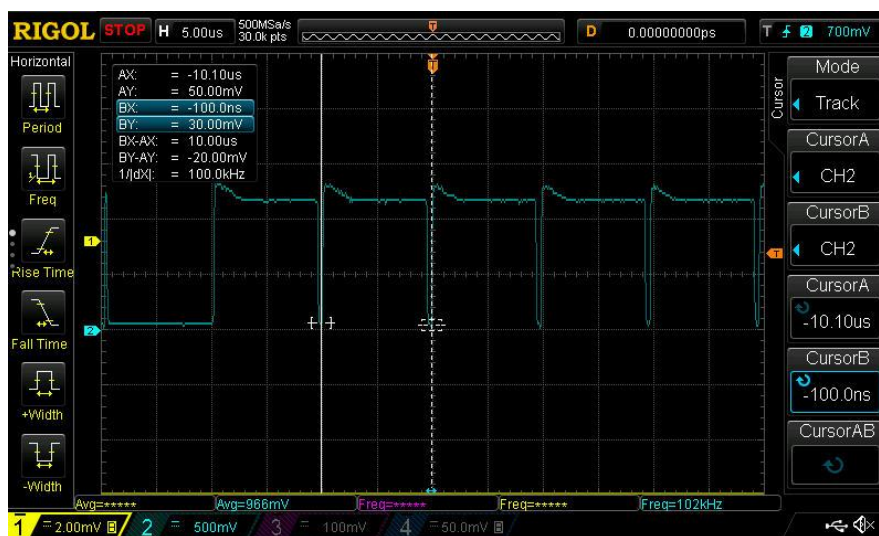
Slika 5.1. Uvećani prikaz upravljačkog signala
