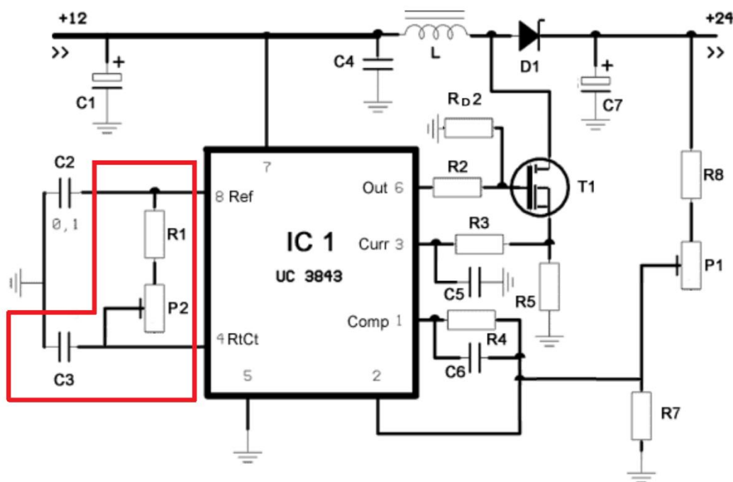
Slika 5.3. Konačne preinake upravljačkog kruga
